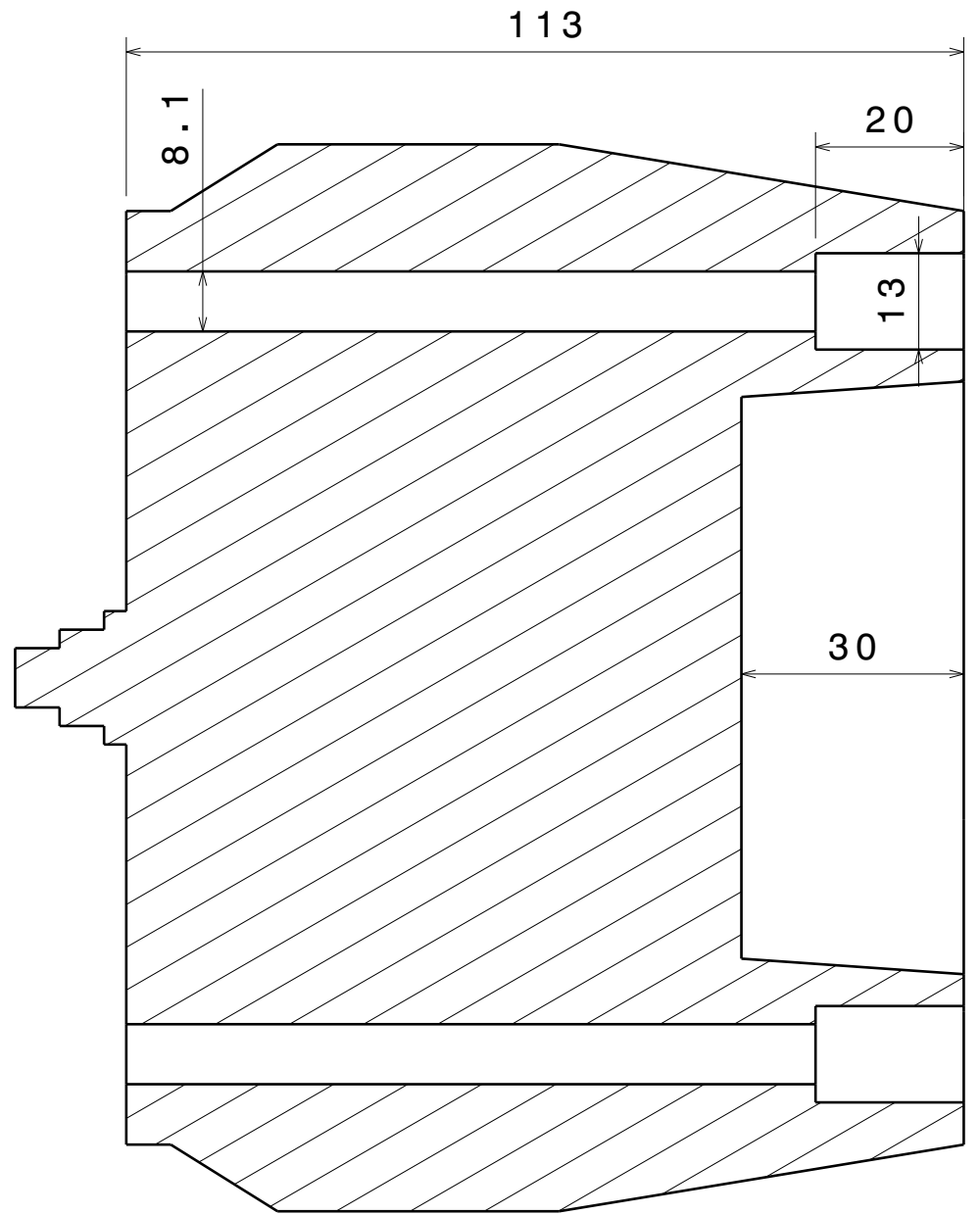
Coupe B-B Echelle : 1:1
